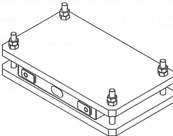
电芯夹具示意图 Steel plate
