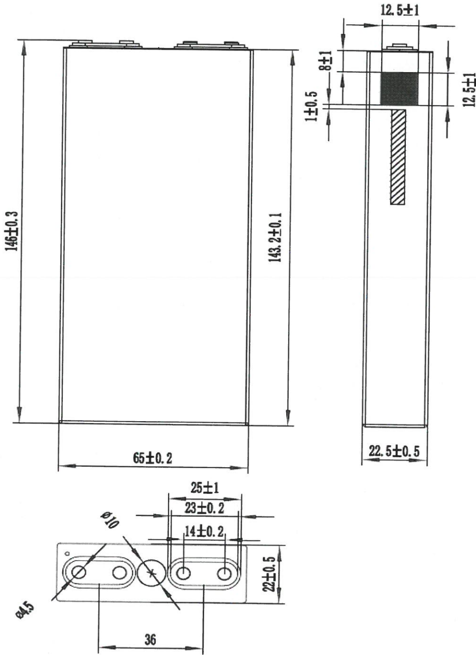
电芯尺寸
