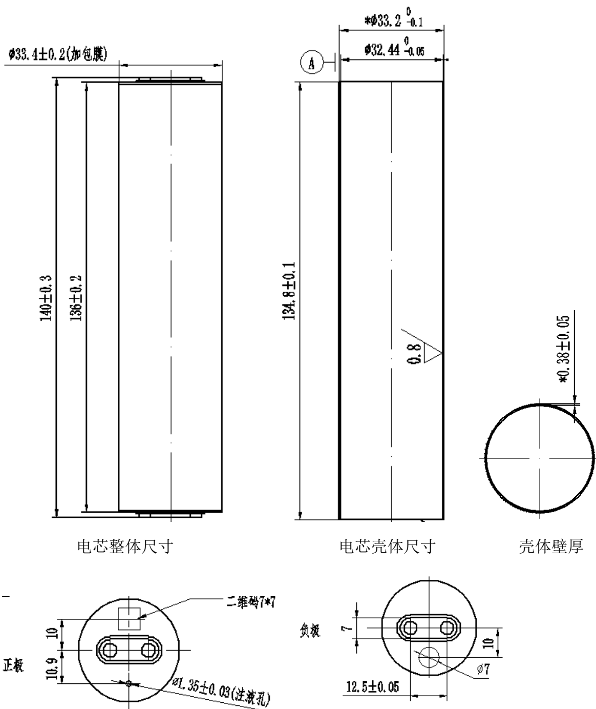
图 A.1 电池尺寸图
